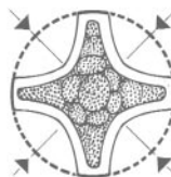
Aggraffatura corretta
